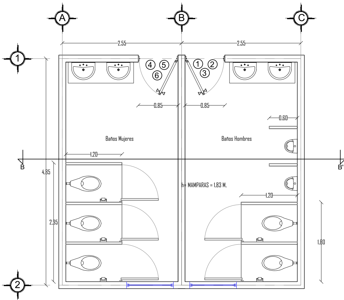
Planta de Baños Planta baja, 1er. Nivel, 2do. Nivel Esc. 1 : 50
