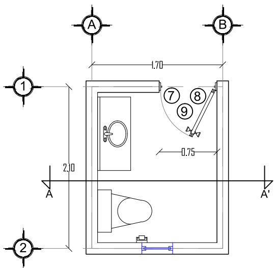
Planta de Baños Individuales Planta baja y 1er Nivel Esc. 1 : 50
